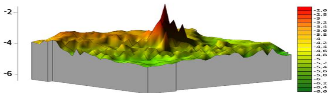
Gambar 3 Sebaran puing-puing rambu penuntun yang telah runtuh
