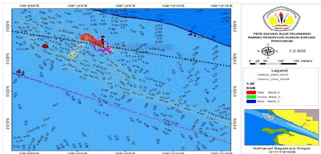
Gambar 5 Peta elevasi kedalaman alur pelayaran
